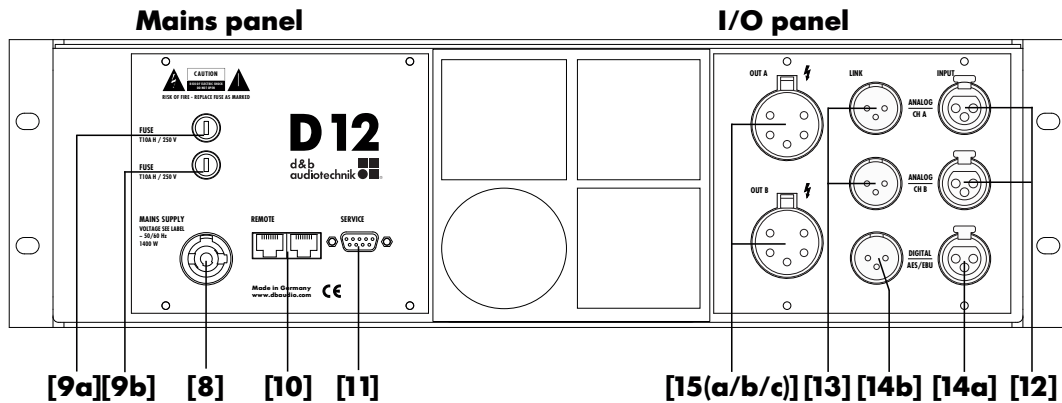
Fig. 8 : connexions D12
