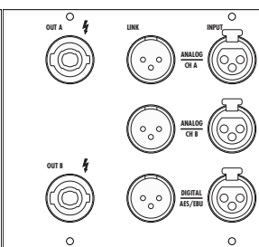
Fig. 28 : panneau I/O des connecteurs NL4 du D12
