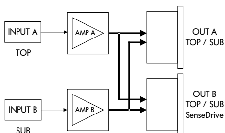
Fig. 18 : routage entrée/sortie du D12 mode mix TOP/SUB avec routage d'entrée standard
