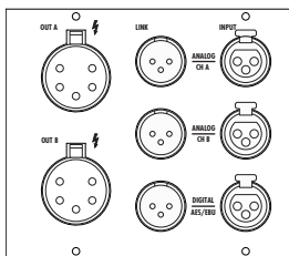
Fig. 12 : panneau I/O du D12
