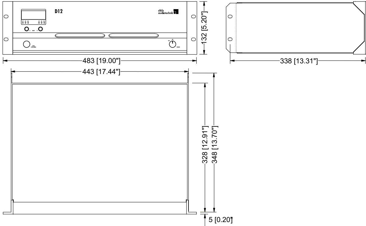
Fig. 25 : dimensions du boîtier du D12 en mm [inch]
