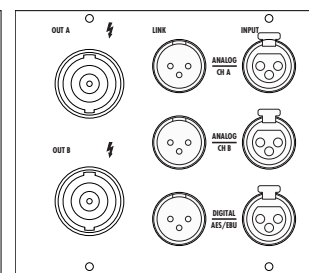
Fig. 29 : panneau I/O des connecteurs NL8 du D12
